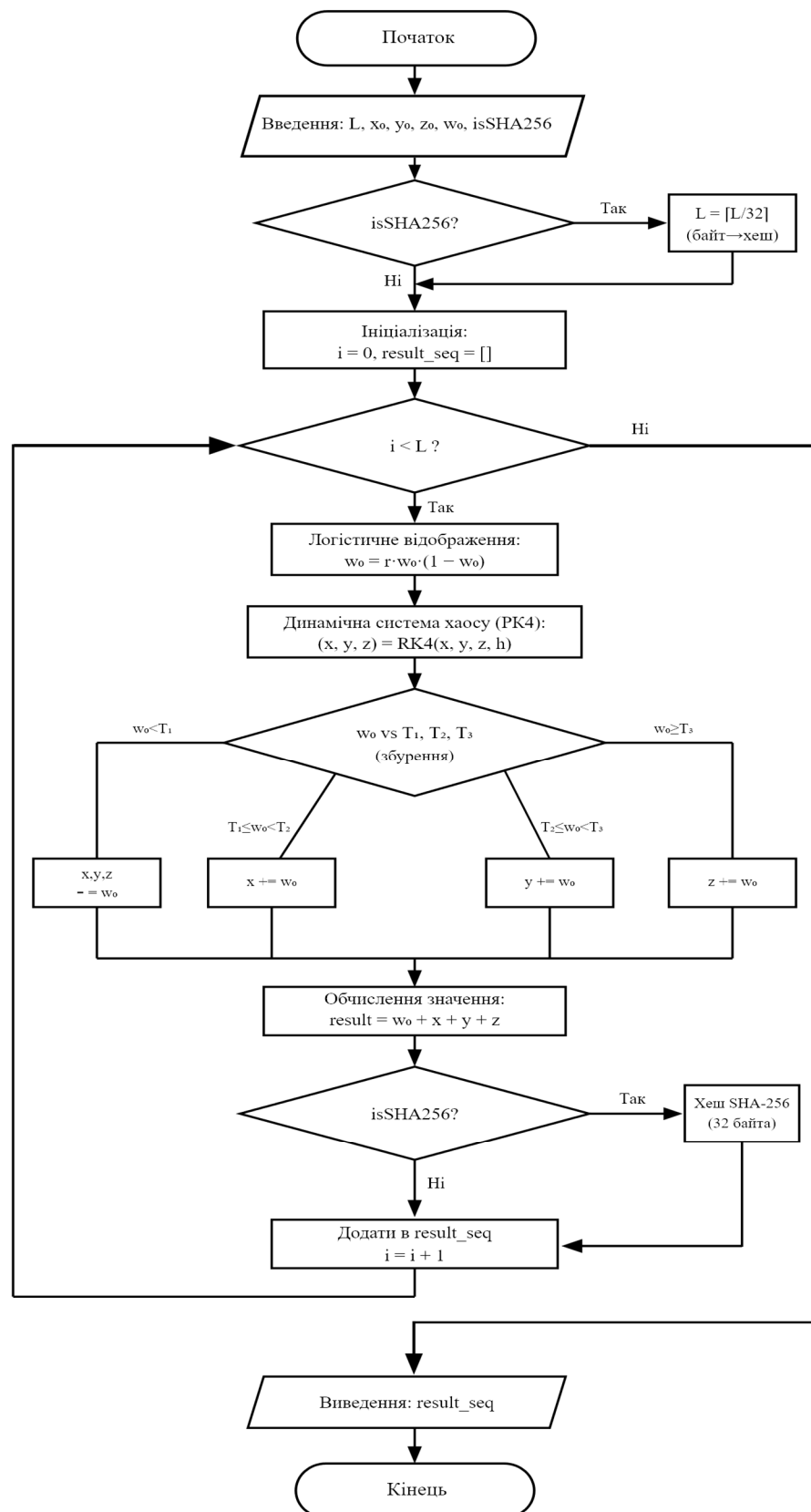
Рисунок 2.1 – Блок-схема генератора псевдохаотичної послідовності
