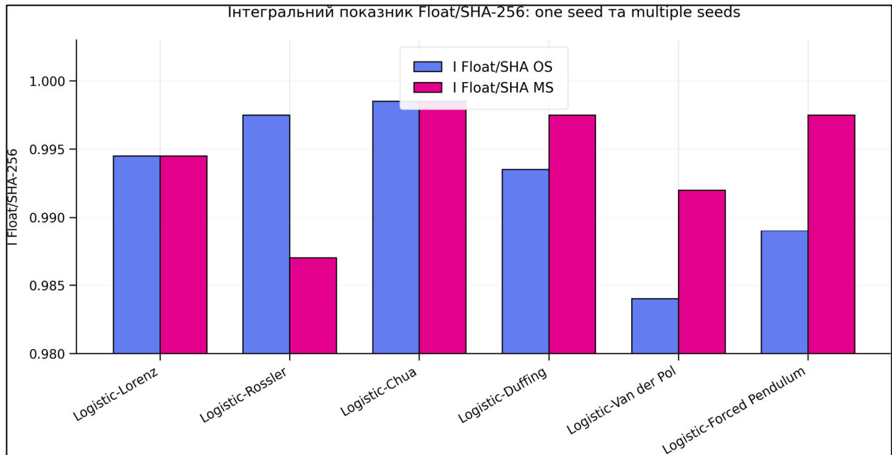
Рисунок 2.14 – Гістограма для I_Float/SHA-256: one seed та multiple seeds
