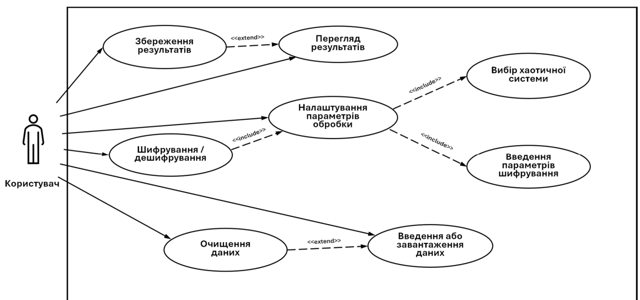
Рисунок 3.1 – Use Case-діаграма демонстраційного застосунку
