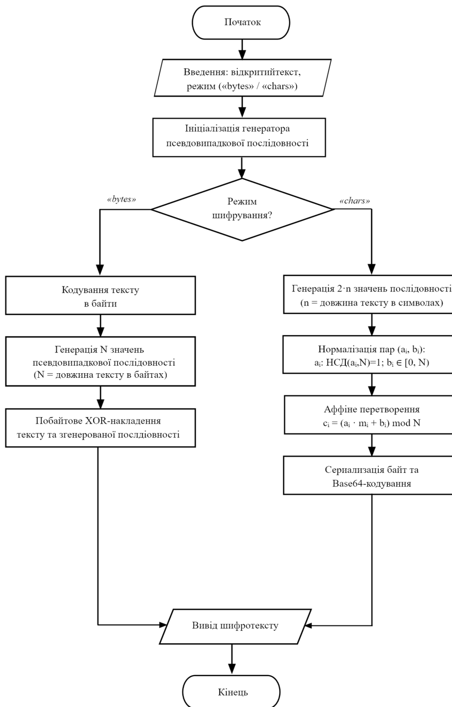
Рисунок 2.3 – Блок-схема алгоритму шифрування тексту
