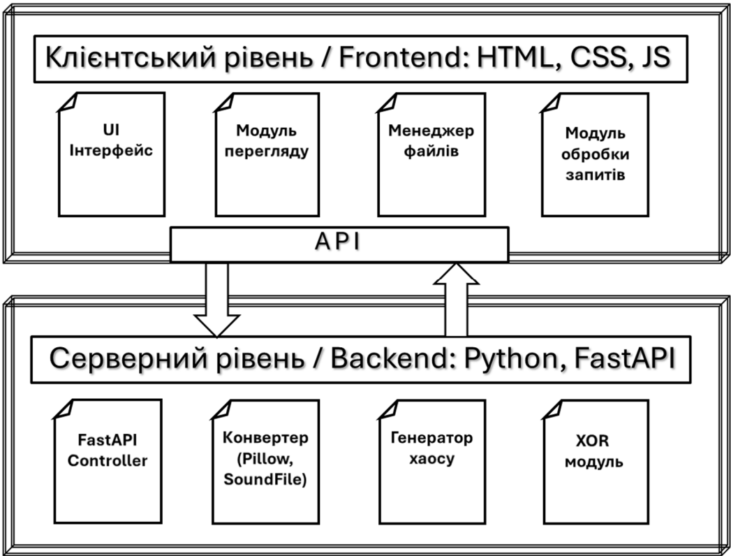
Рисунок 3.2 – Схема архітектури демонстраційного застосунку
