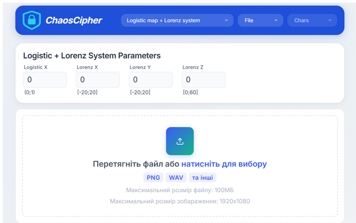
Рисунок 3.3 – Головна сторінка клієнтської частини застосунку
